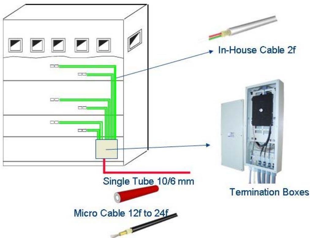
Σχ.27.: Σημείο εισόδου σε πολυκατοικία (περίπτωση 1)
