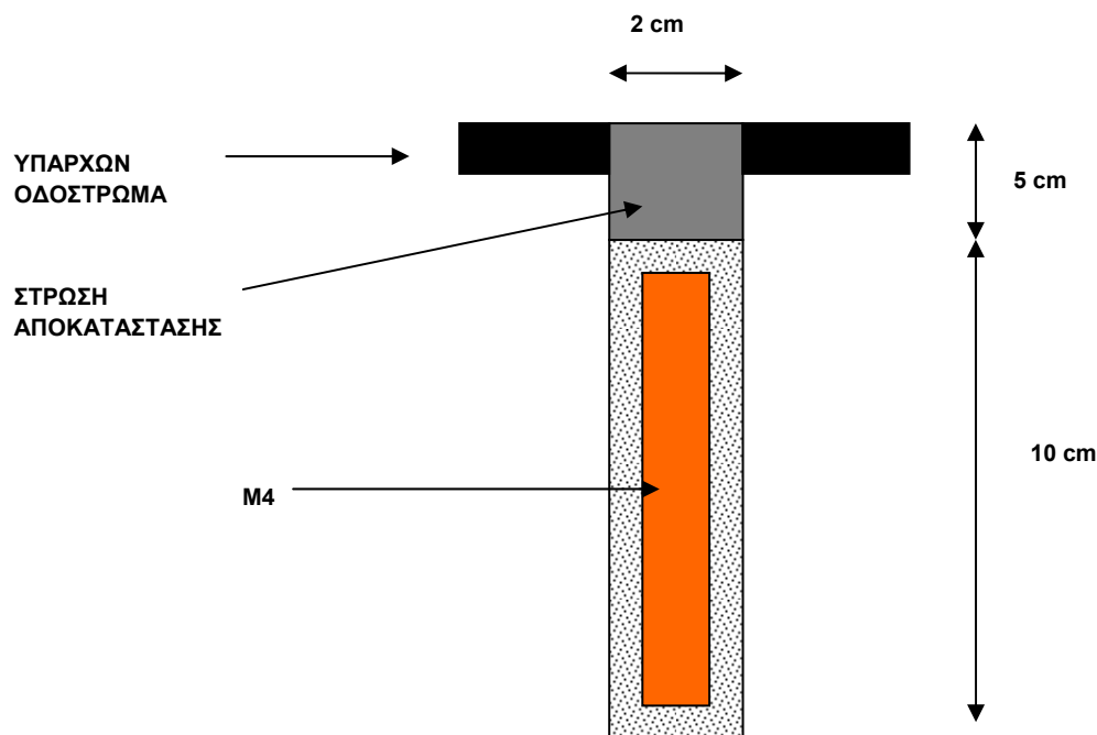
Σχ.16.: Τυπική τομή Χάνδακα X3
