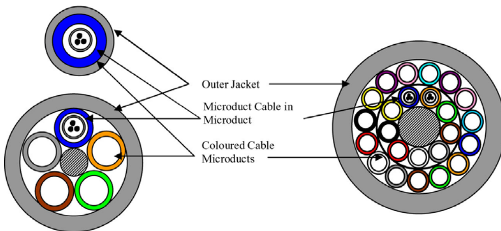
Σχ.20.: Μικροσωλήνας προστατευόμενου καλωδίου με ενσωματωμένο σφιχτό εξωτερικό σωλήνα
