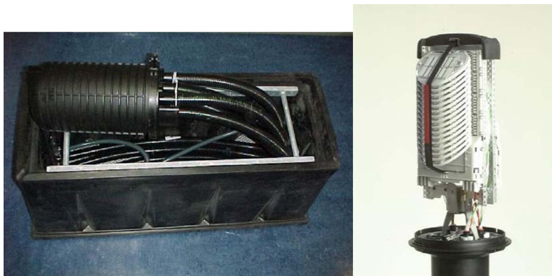
Σχ.22.: Διατάξεις συγκόλλησης Ινών
