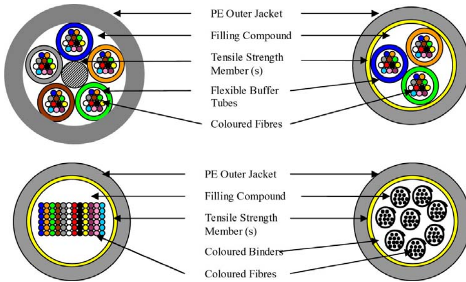
Σχ.18.: Καλώδια μικροσωλήνων οπτικών ινών
