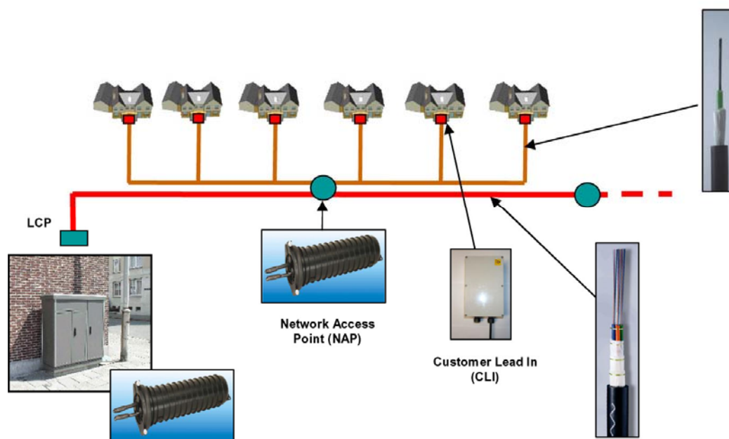
Σχ.1.: Συμβατική Υποδομή με Σωλήνες
