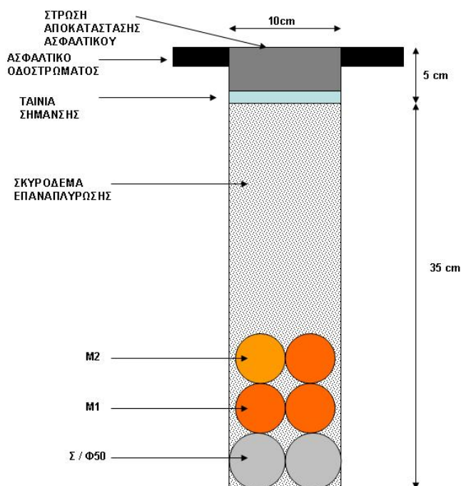
Σχ.14.: Τυπική τομή Χάνδακα X1
