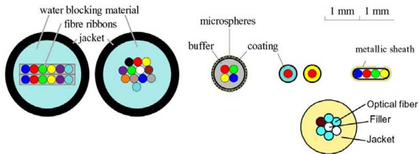
Σχ.19.: Μονάδες οπτικής ίνας
