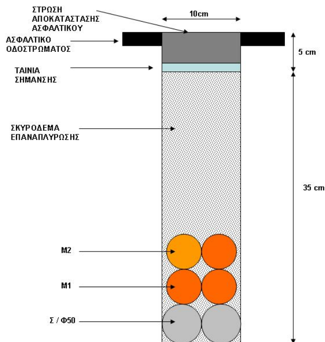
Σχ.14.: Τυπική τομή Τάφρου X1
